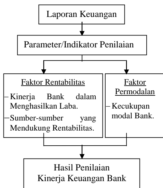
Gambar 1 Kerangka Berpikir
